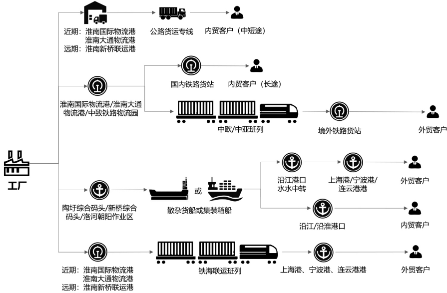
图 4-3 高端装备物流组织方案
