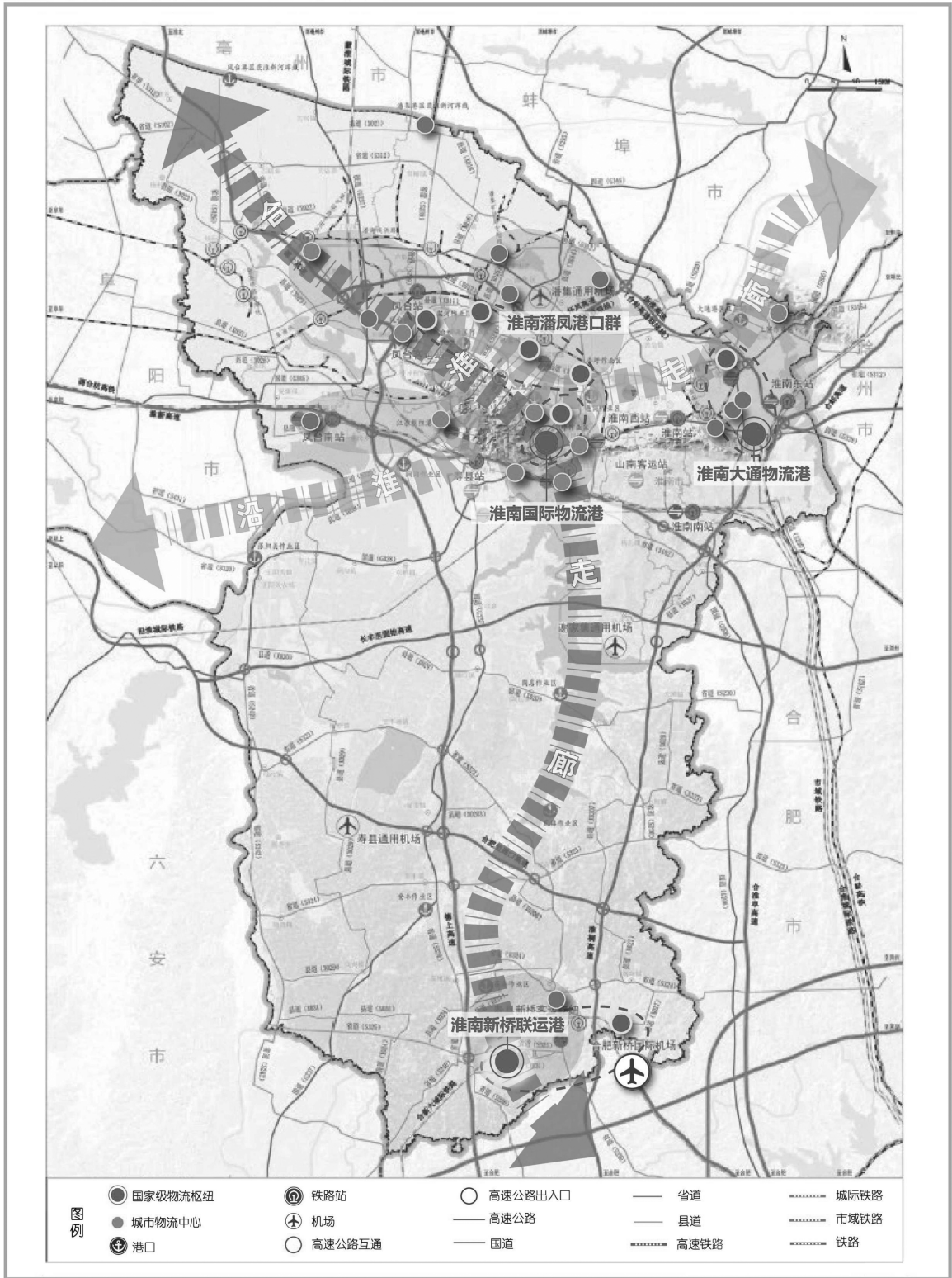
图 3-1 淮南市物流枢纽布局图
