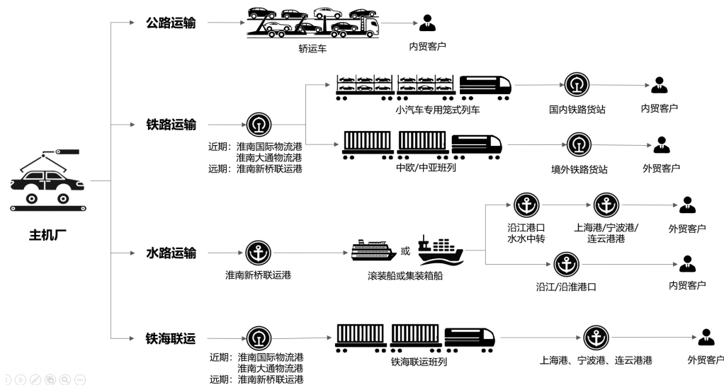
图 4-1 新能源汽车物流组织方案
